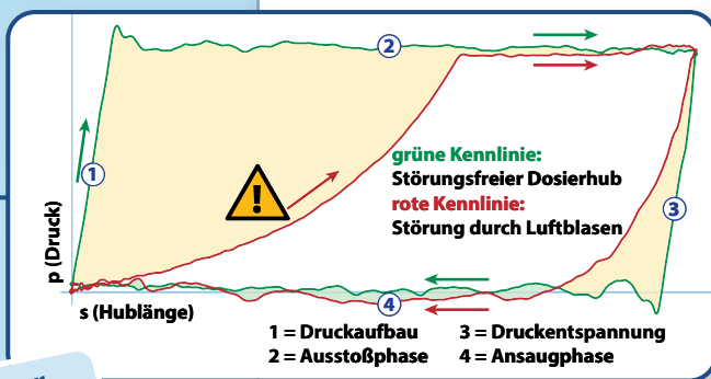
Indikator- diagramm
